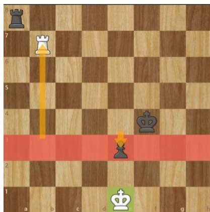
Diagram 2 – Eksempel på trin 2 af en almindelig Philidor-stilling.
