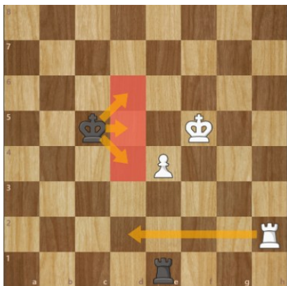
Diagram 8 – Eksempel på trin 1 af en almindelig Lucena-stilling
