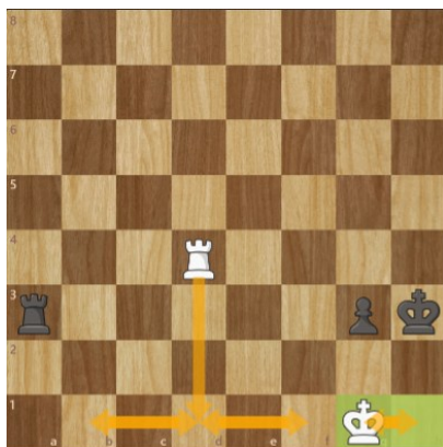
Diagram 4 – Eksempel på baglinjeforsvar mod g-bonde.
