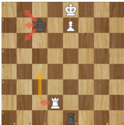
Diagram 11 – Eksempel på trin 4 i en almindelig Lucena-stilling. Sort er i trækket, men kan intet stille op.
