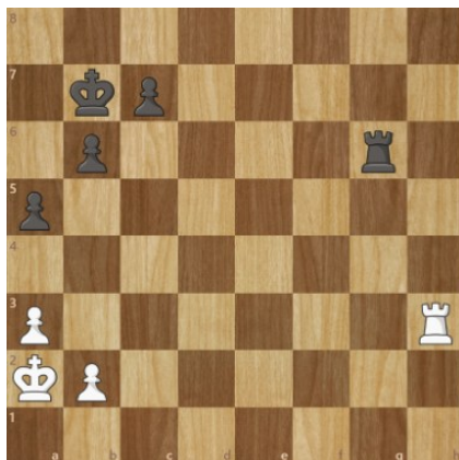
Diagram 6 – Et klassisk eksempel på et remis tårnslutspil, hvor hvid er en bonde nede.
