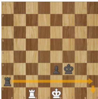
Diagram 5 – Eksempel på forfejlet baglinjeforsvar, da modstanderens bonde er en e-bonde – Sort har mat på 13. Hvid skulle have brugt Philidor-stillingen tidligere i partiet.
