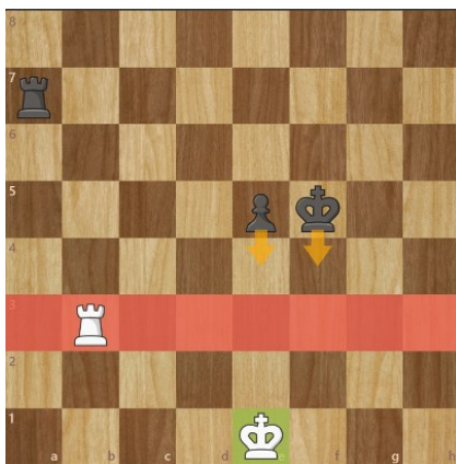
Diagram 1 – Eksempel på trin 1 af en almindelig Philidor-stilling.
